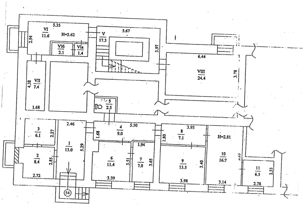
ПОВЕРХ цокол. ЛІТЕР "А"
